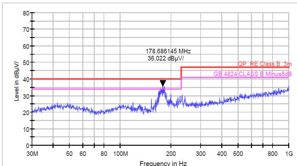
图 3-6 辐射测试水平方向
